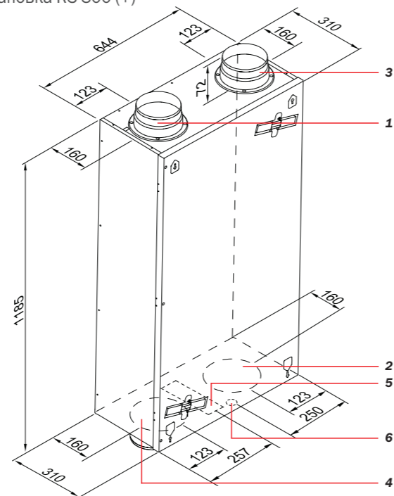
Установка RS 300 (+)
